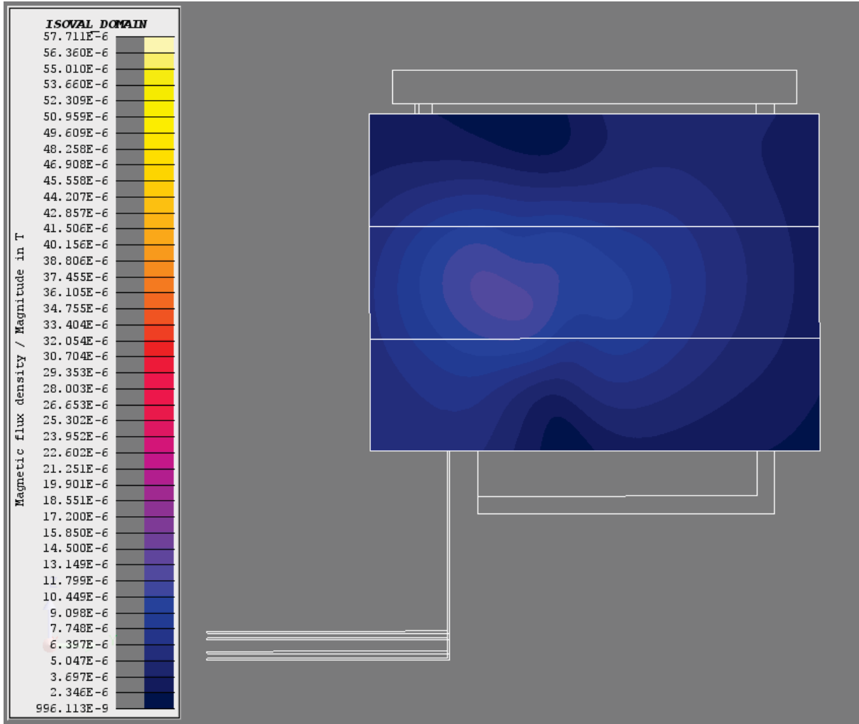
Figura 84. Densidad de flujo magnético (B[T] = Magnitud B) en el panel derecho (3L [Semi]).
