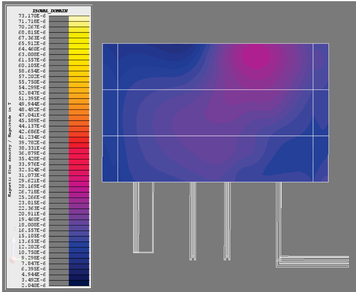
Figura 48. Densidad de flujo magnético (B[T] = Magnitud B) en el panel derecho (2L+1T [Semi]).
