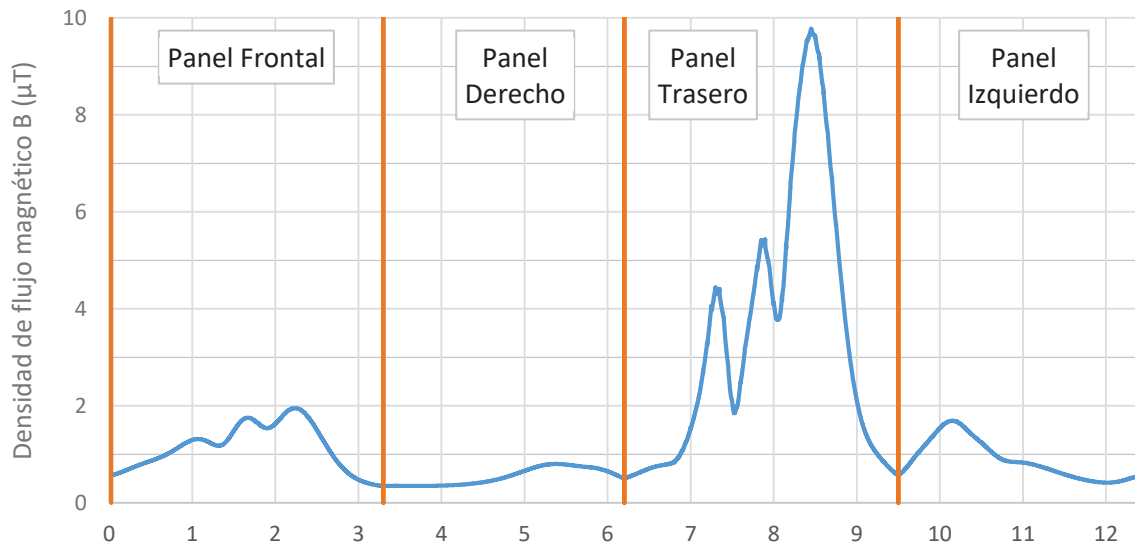
Figura 75. Densidad de flujo magnético (B[T] = Magnitud B) en envoltorio situada a 0,5 metros (3L [Sup]).
