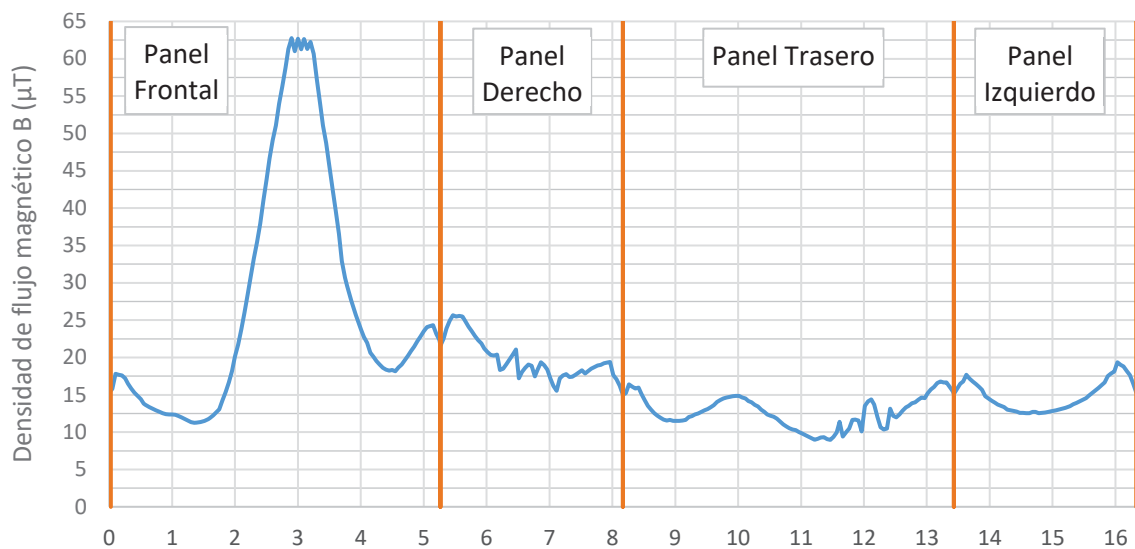
Figura 10. Densidad de flujo magnético ( B[T] = \text{Magnitud } B ) en envoltorio situada a 1 metro ( 2L+1T [Sup]).
