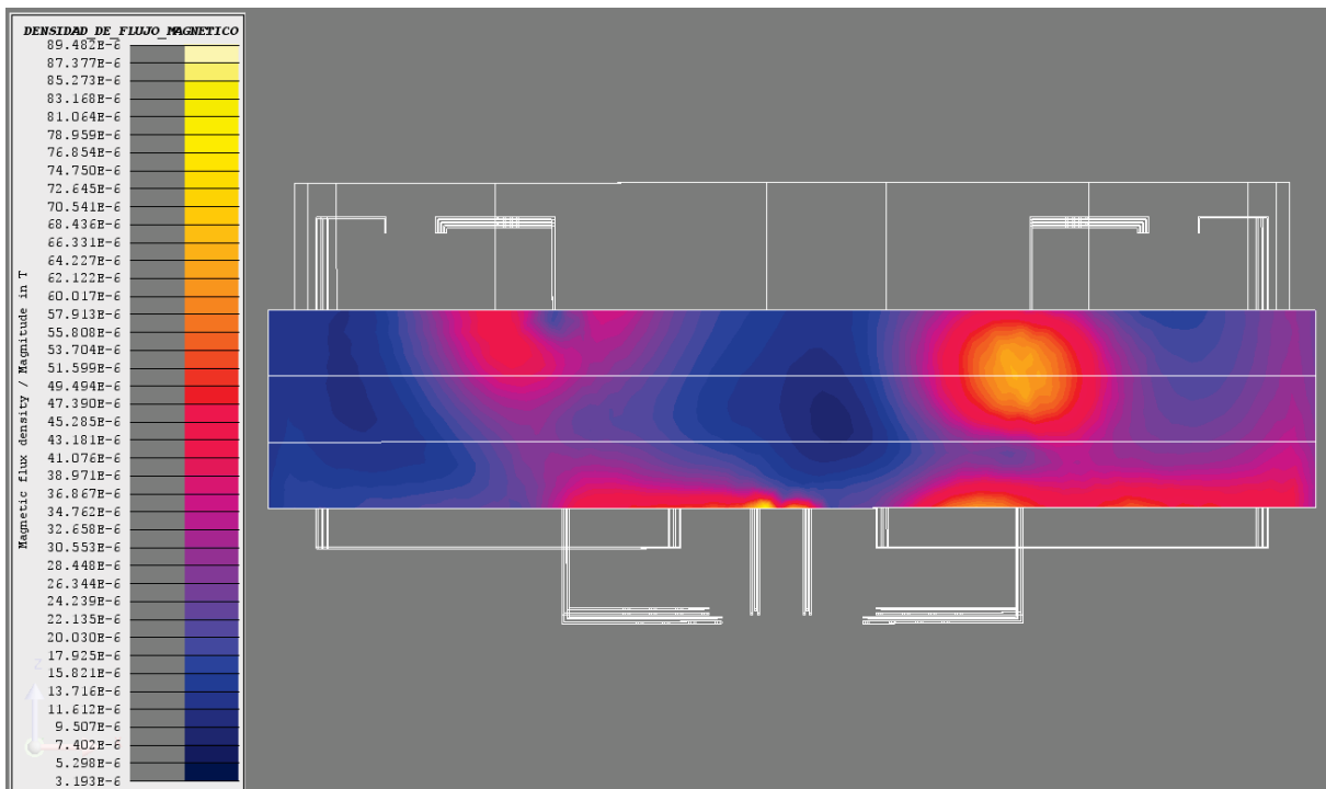
Figura 16. Densidad de flujo magnético [B[T] = \text{Magnitud } B] en el panel frontal (2L+2T \text{ [Sup]}) .
