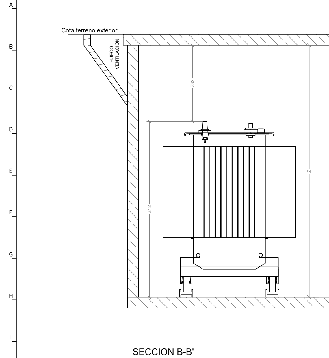
SECCION B-B'
