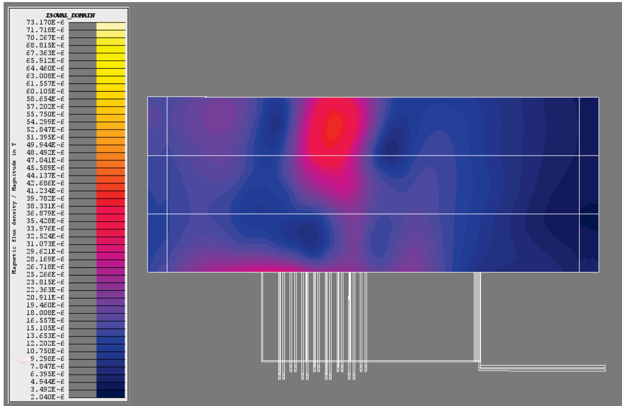
Figura 49. Densidad de flujo magnético ( B[T] = \text{Magnitud } B ) en el panel trasero (2L+1T [Semi]).
