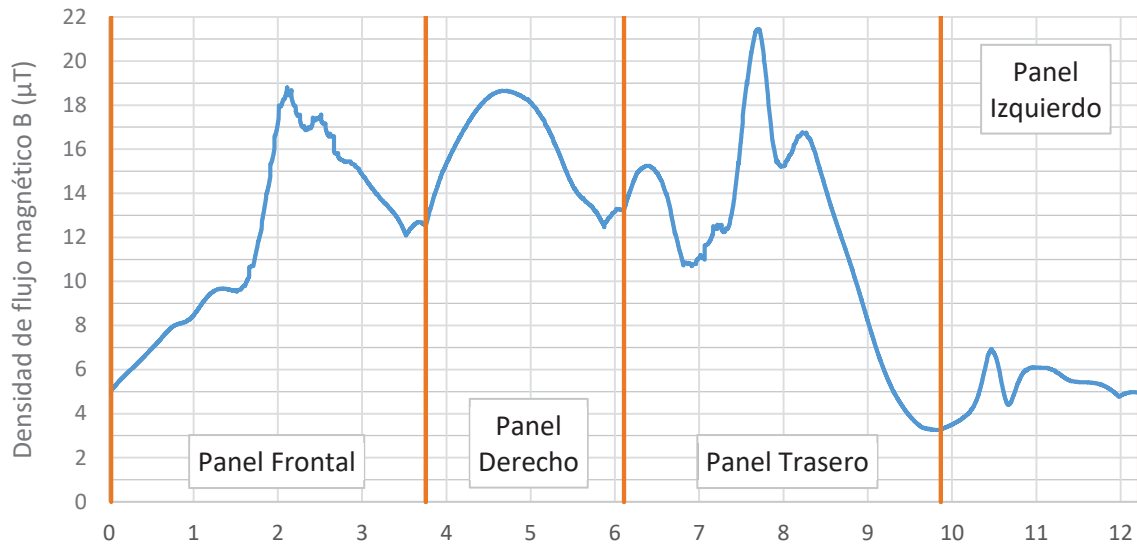
Figura 51. Densidad de flujo magnético ( B[T] = \text{Magnitud } B ) en envoltorio situada a 0,5 metros (2L+1T [Semi]).
