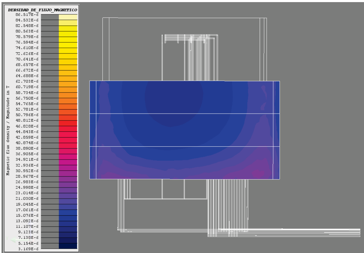
Figura 8. Densidad de flujo magnético (B[T] = Magnitud B) en el panel izquierdo (2L+1T [Sup]).
