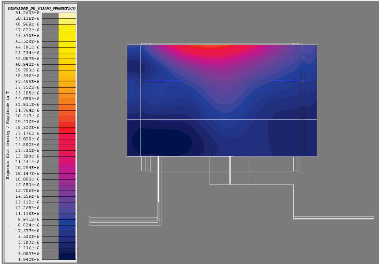
Figura 61. Densidad de flujo magnético (B[T] = Magnitud B) en el panel trasero (1T [Rural]).
