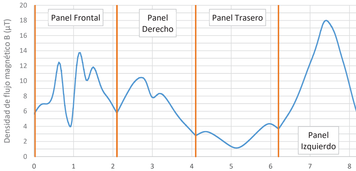
Figura 87. Densidad de flujo magnético ( B[T] = \text{Magnitud } B ) en envoltente situada a 0,5 metros (3L [Semi]).
