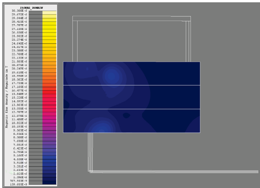
Figura 74. Densidad de flujo magnético ( B[T] = \text{Magnitud } B ) en el panel izquierdo (3L [Sup]).
