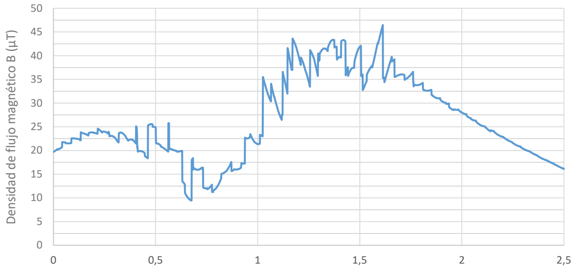
Figura 40. Densidad de flujo magnético ( B[T] = \text{Magnitud } B ) en línea 2 (2L+2T [SUB]).
