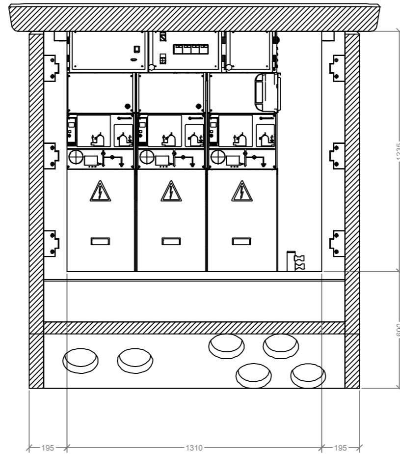
ALZADO PRINCIPAL SIN PUERTAS
