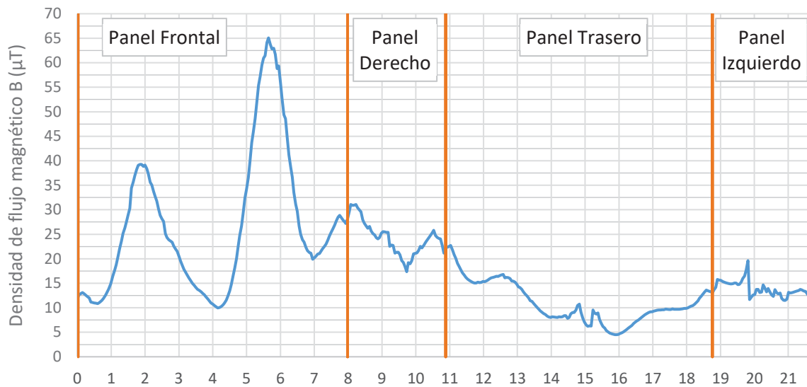
Figura 21. Densidad de flujo magnético ( B[T] = \text{Magnitud } B ) en envolvente situada a 1 metro ( 2L+2T [Sup]).
