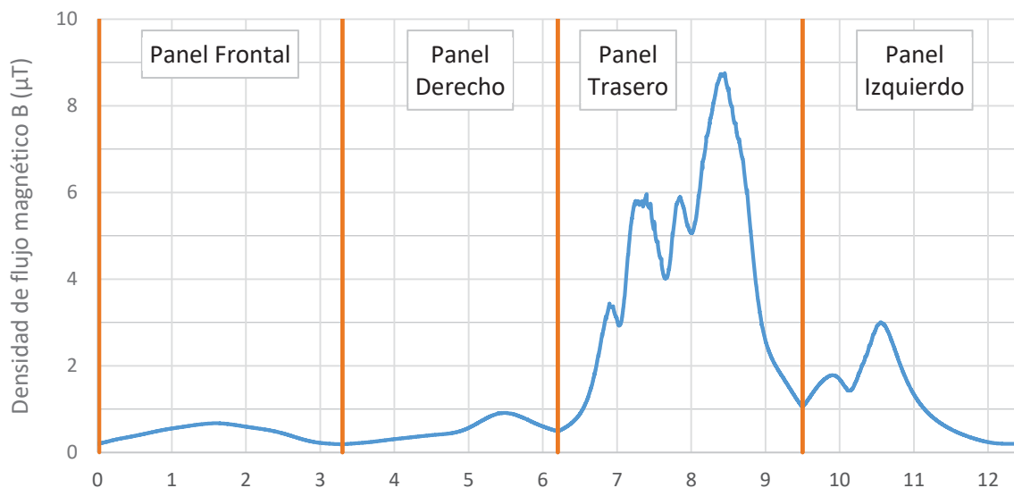
Figura 76. Densidad de flujo magnético (B[T] = Magnitud B) en envoltorio situada a 1 metro (3L [Sup]).
