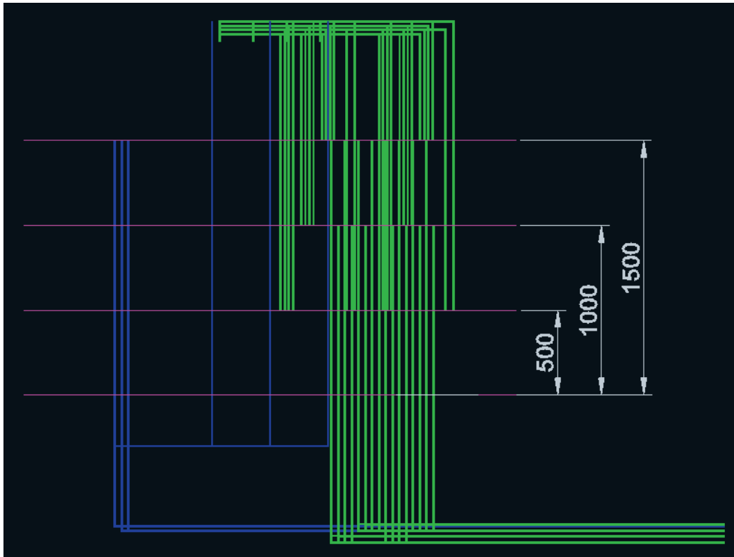
Figura 14. Vista en perfil de la instalación (2L+2T [Sup]) (cotas en mm).
