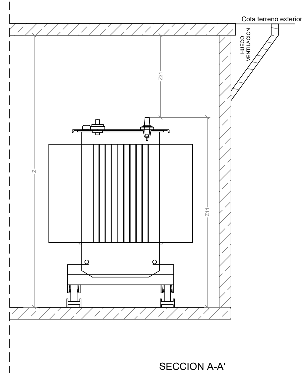
SECCION A-A'
