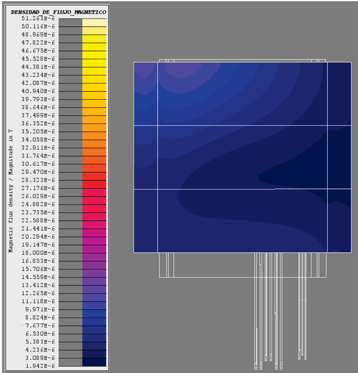
Figura 62. Densidad de flujo magnético (B[T] = Magnitud B) en el panel izquierdo (1T [Rural]).
