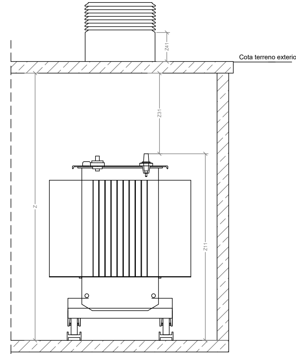
SECCION A-A'
