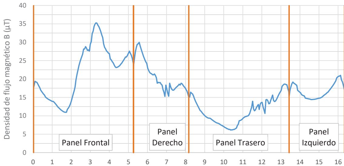
Figura 9. Densidad de flujo magnético ( B[T] = \text{Magnitud } B ) en envoltorio situada a 0,5 metros ( 2L+1T [Sup]).
