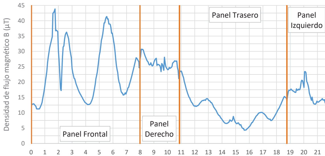
Figura 22. Densidad de flujo magnético ( B[T] = \text{Magnitud } B ) en envolvente situada a 1,5 metros (2L+2T [Sup]).
