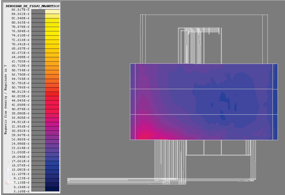
Figura 6. Densidad de flujo magnético ( B[T] = \text{Magnitud } B ) en el panel derecho (2L+1T [Sup]).
