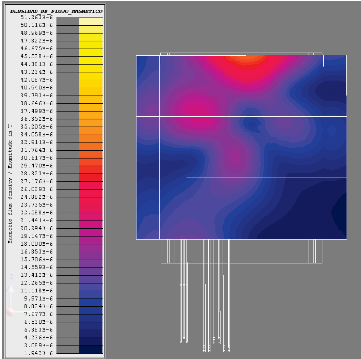
Figura 60. Densidad de flujo magnético (B[T] = Magnitud B) en el panel derecho (1T [Rural]).
