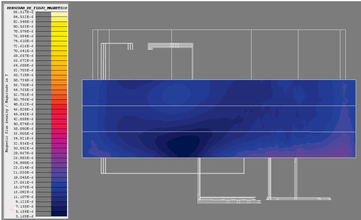
Figura 7. Densidad de flujo magnético (B[T] = Magnitud B) en el panel trasero (2L+1T [Sup]).
