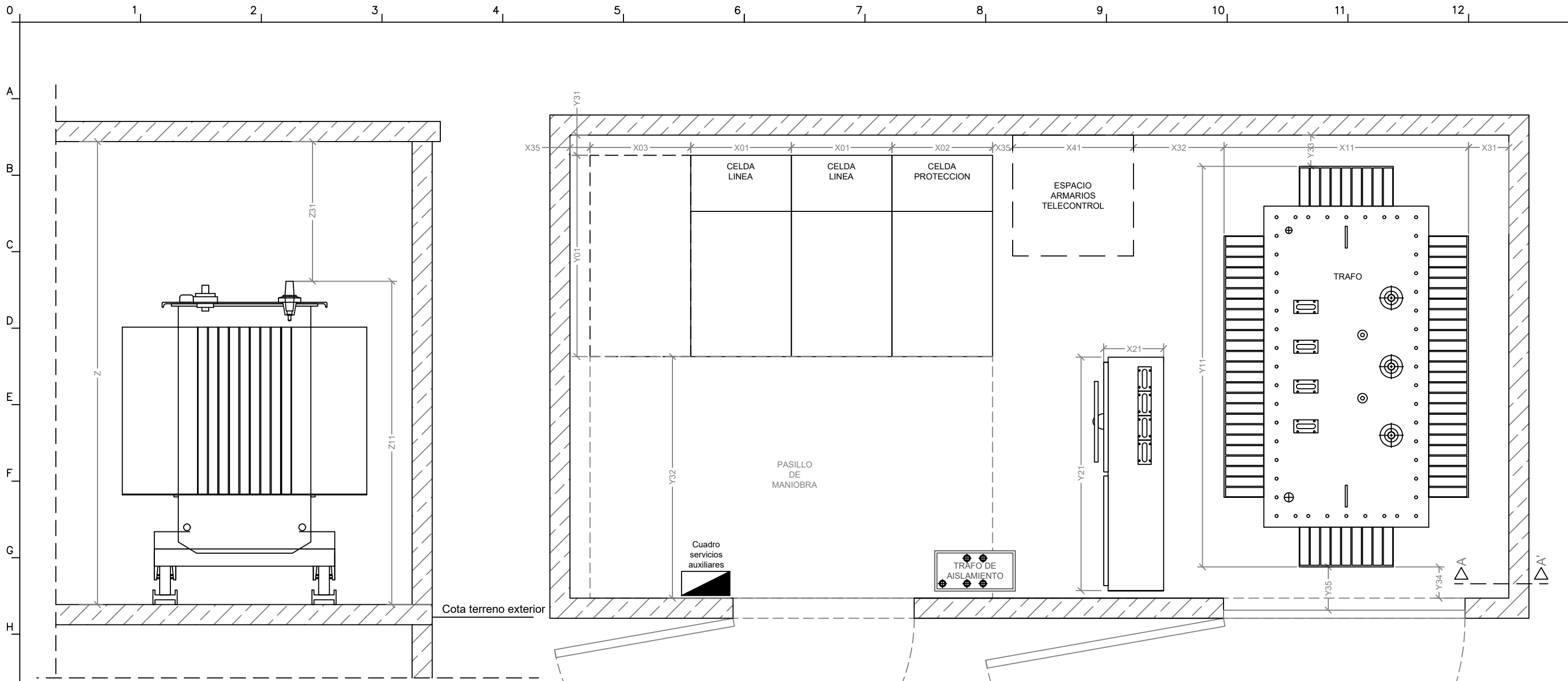
SECCION A-A'
