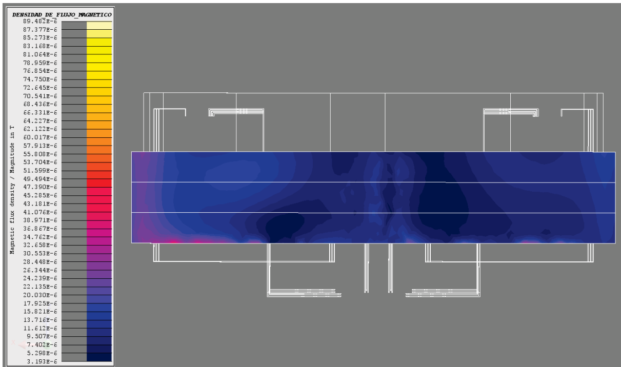
Figura 18. Densidad de flujo magnético ( B[T] = \text{Magnitud } B ) en el panel trasero (2L+2T [Sup]).
