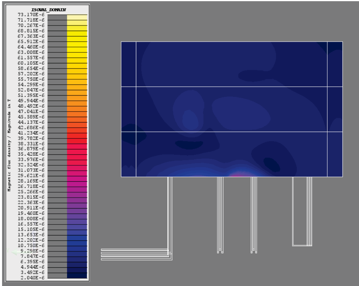
Figura 50. Densidad de flujo magnético ( B[T] = \text{Magnitud } B ) en el panel izquierdo ( 2L+1T [Semi]).
