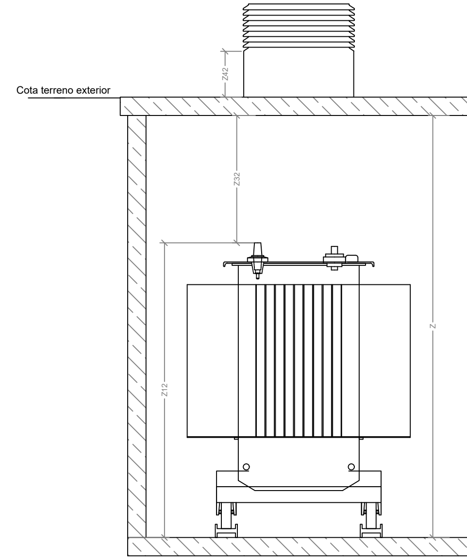
SECCION A-A'
