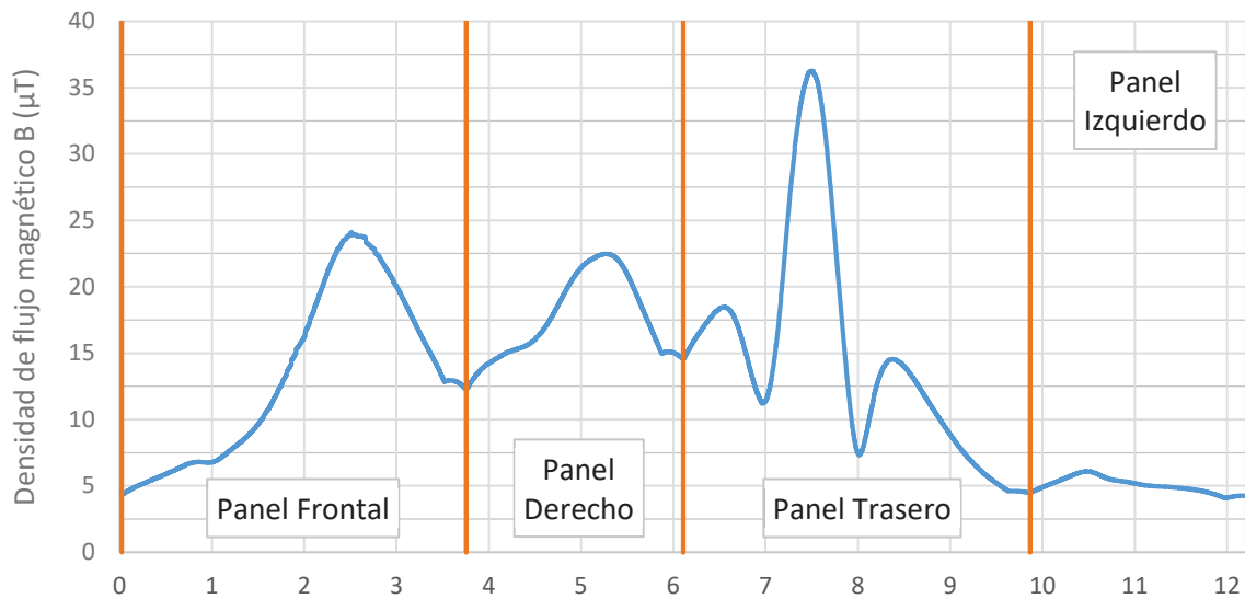
Figura 52. Densidad de flujo magnético ( B[T] = \text{Magnitud } B ) en envoltorio situada a 1 metro (2L+1T [Semi]).
